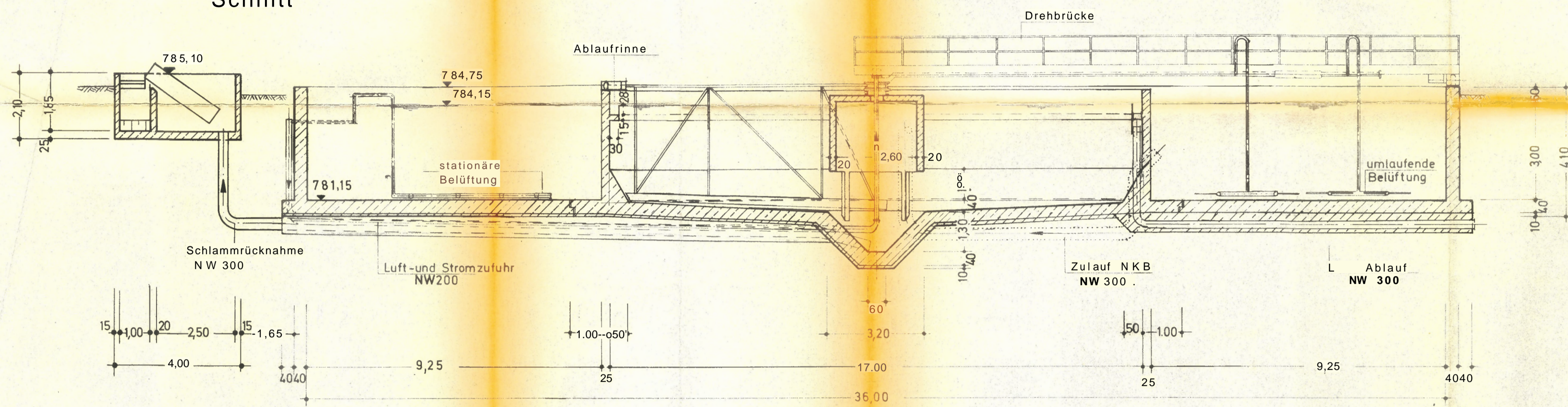
Schnitt
